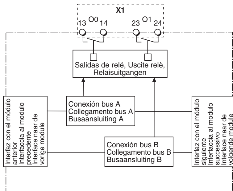
Fig. 1: Schema connessioni
