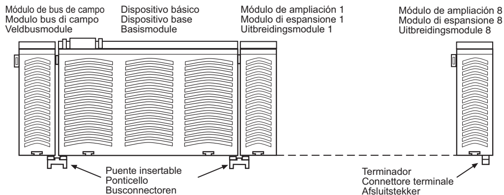
Fig. 2: Basisgerät und Erweiterungsmodul verbinden
